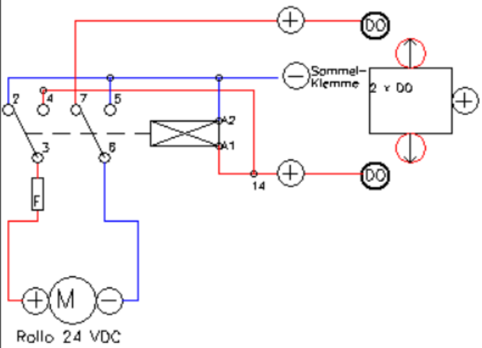
Beschaltung Rollos in SPS Schrank über Relais
