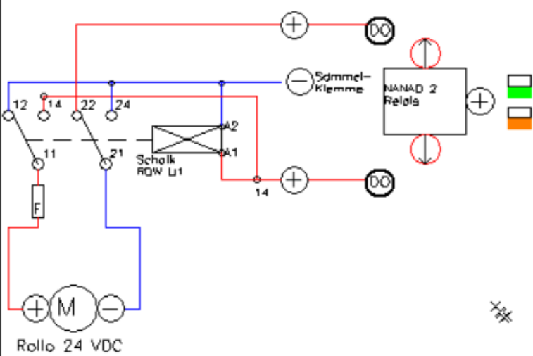
Beschaltung Rollos in SPS Schrank über Nano2 Tree Relais
